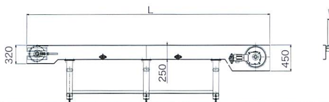
■断面詳細図
