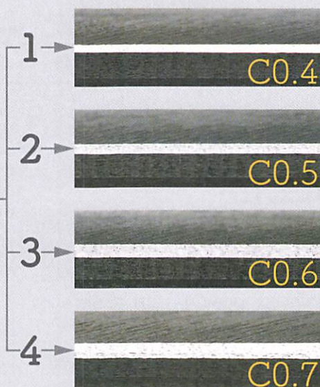
バリ取り例
