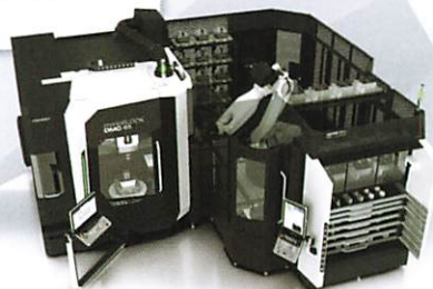
ワーク&パレット搬送システム MATRIS WPH 210
